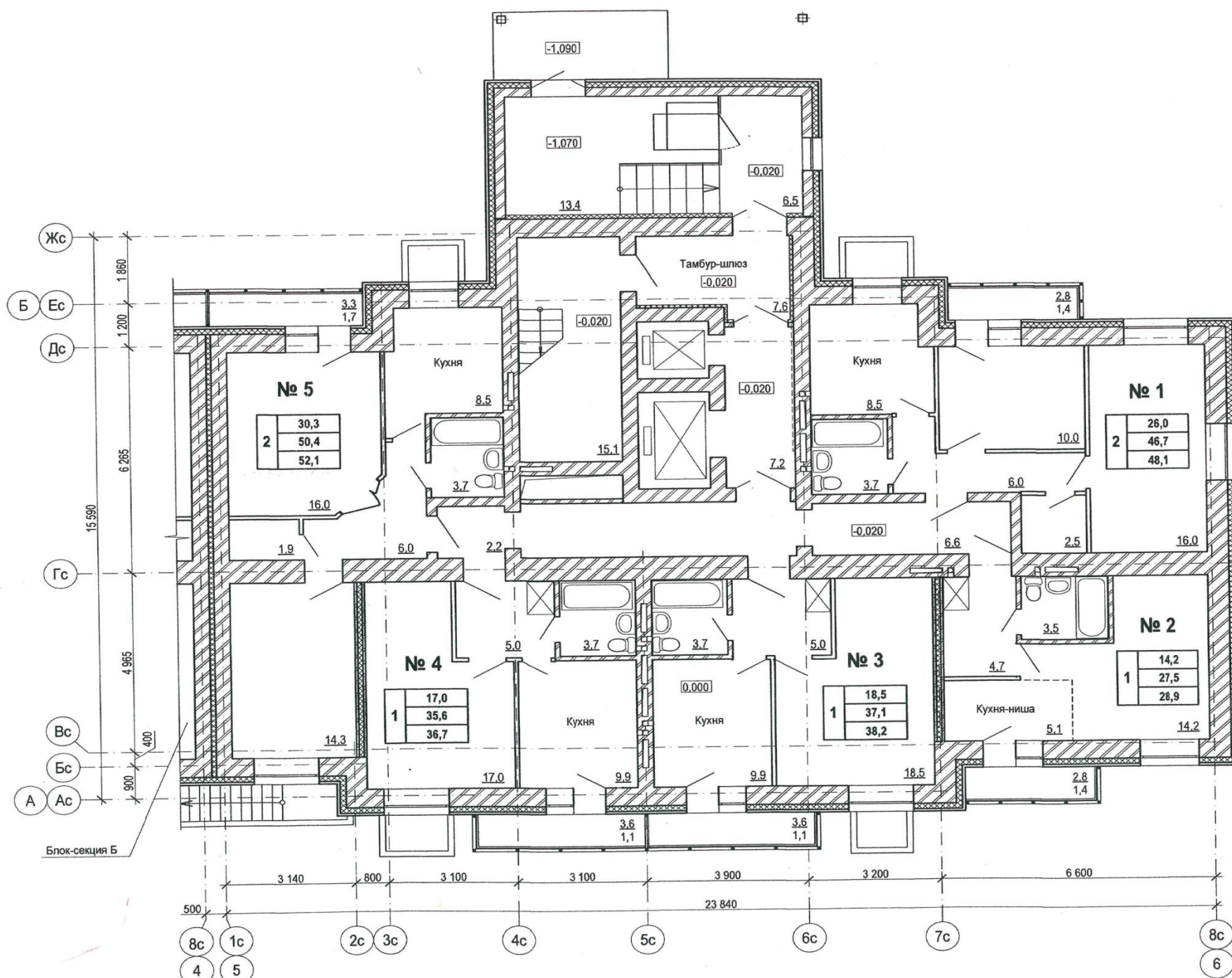
163 квартирный жилой дом. План первого этажа.
